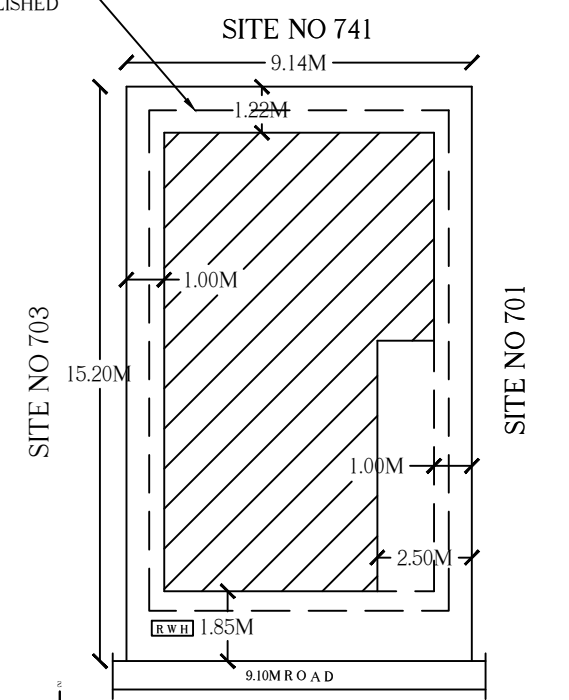
SITE PLAN 1:200
